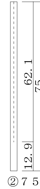
防鳩ルーバー（羽部分断面）S = 1 / 1
