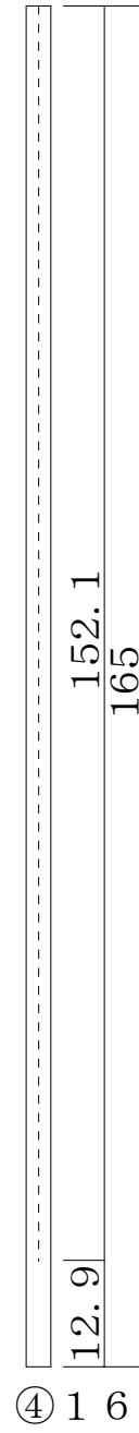
防鳩ルーバー（羽部分断面）S = 1 / 1
