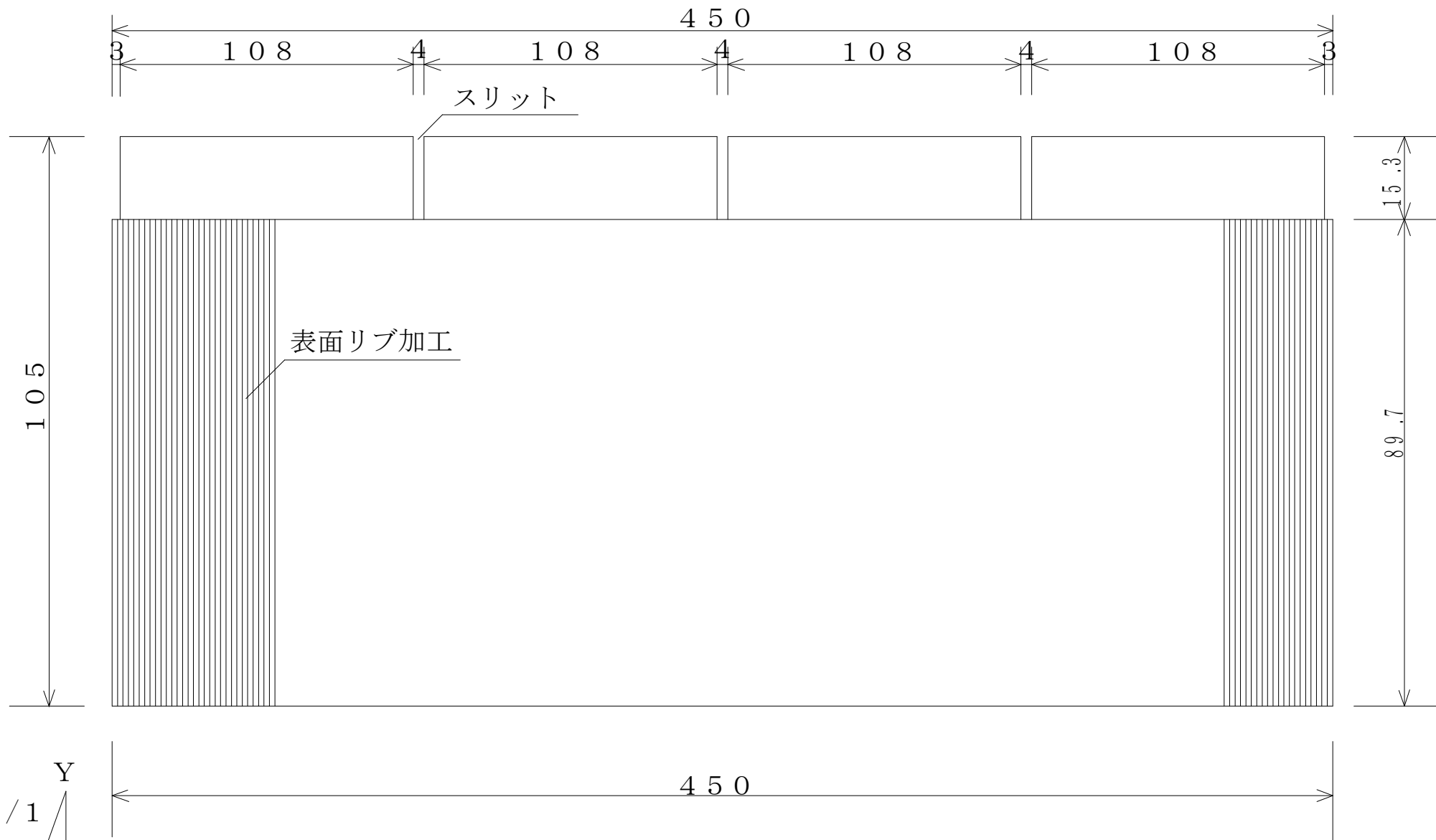
防鳩ルーバー（羽部分正面）X方向 1 / 2 Y方向 1 / 1
