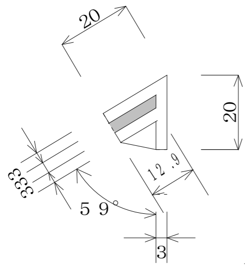
防鳩ルーバー (本体部断面) 20mmタイプ S=1/1
